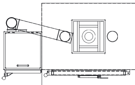
nebenstehender Raucherzeuger external smoke generator
